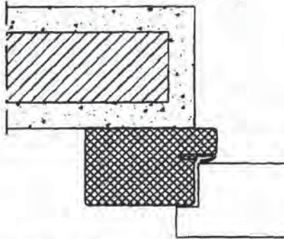
Holzblock zarge 45x75mm zwischen der Wandöffnung
