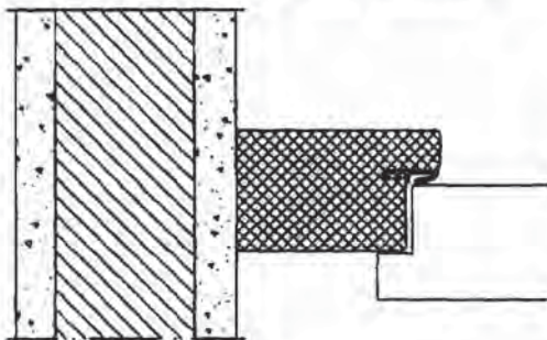
Holzblock zarge 45x75mm zwischen der Wandöffnung
