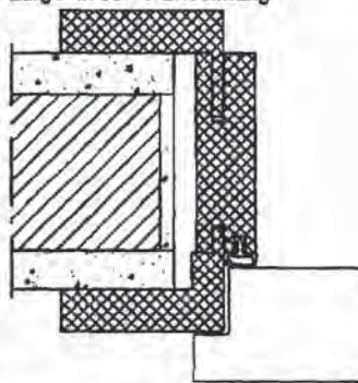
Holzblock zarge in der Wandöffnung
