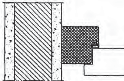
Holzblock zarge 58x58mm zwischen der Wandöffnung
