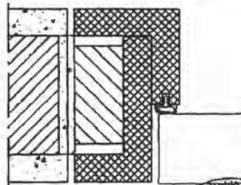
Holzblock zarge in der Wandöffnung
