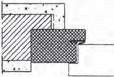
Holzblock zarge 45x75mm in der Wandöffnung (Prüfbericht Nr. 22-16/00E)
