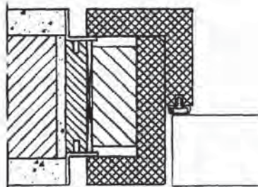
Holzblock zarge in der Wandöffnung
